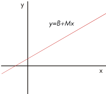
Lineares Kurvenanpassungsmodell
