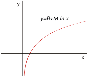
Logarithmisches Kurvenanpassungsmodell
