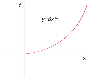
Potenz-Kurvenanpassungsmodell
