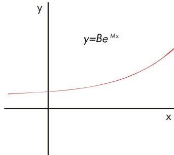
Exponentielles Kurvenanpassungsmodell
